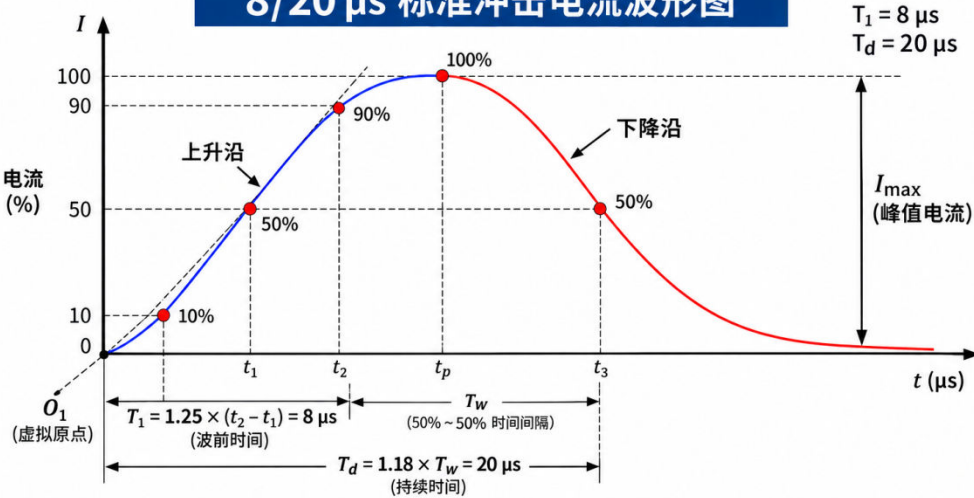
8/20 μs 标准冲击电流波形图
