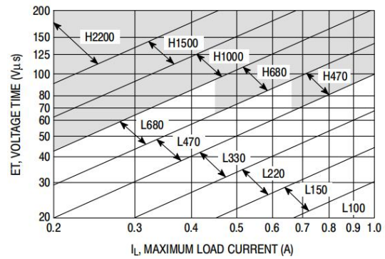
Figure 20. XLM2575-Adj
