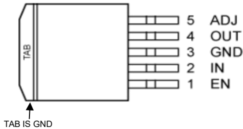
TO-263-5
