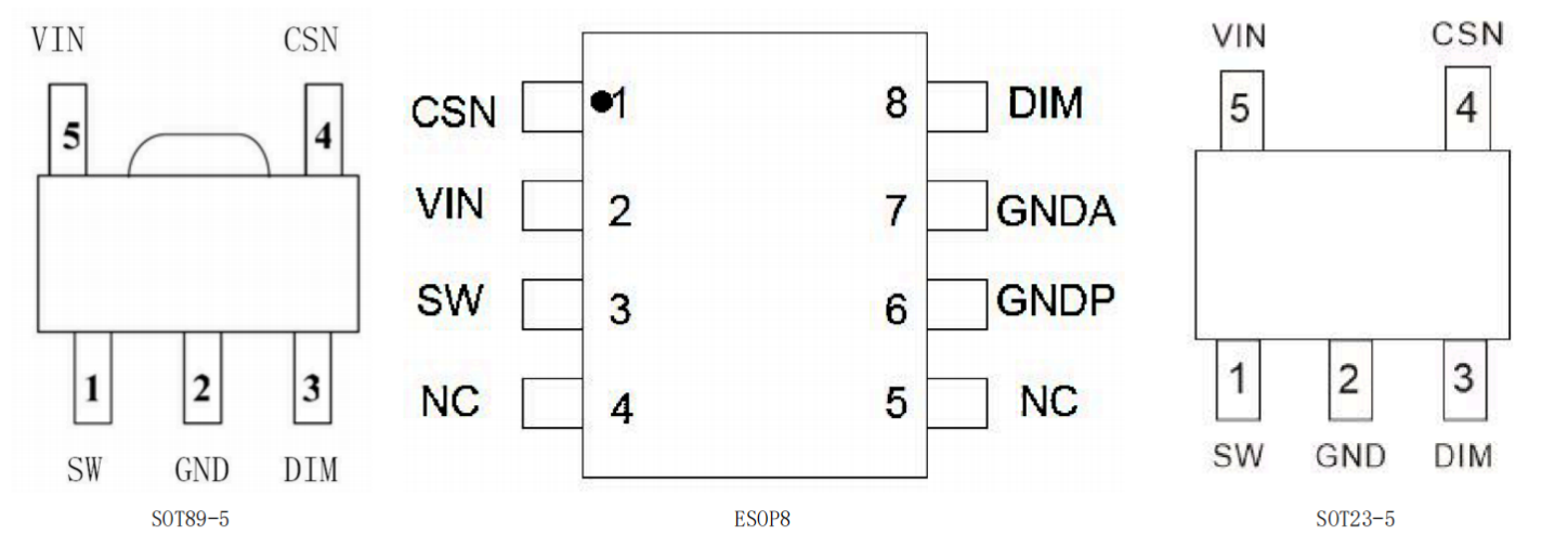
管脚排列图：
