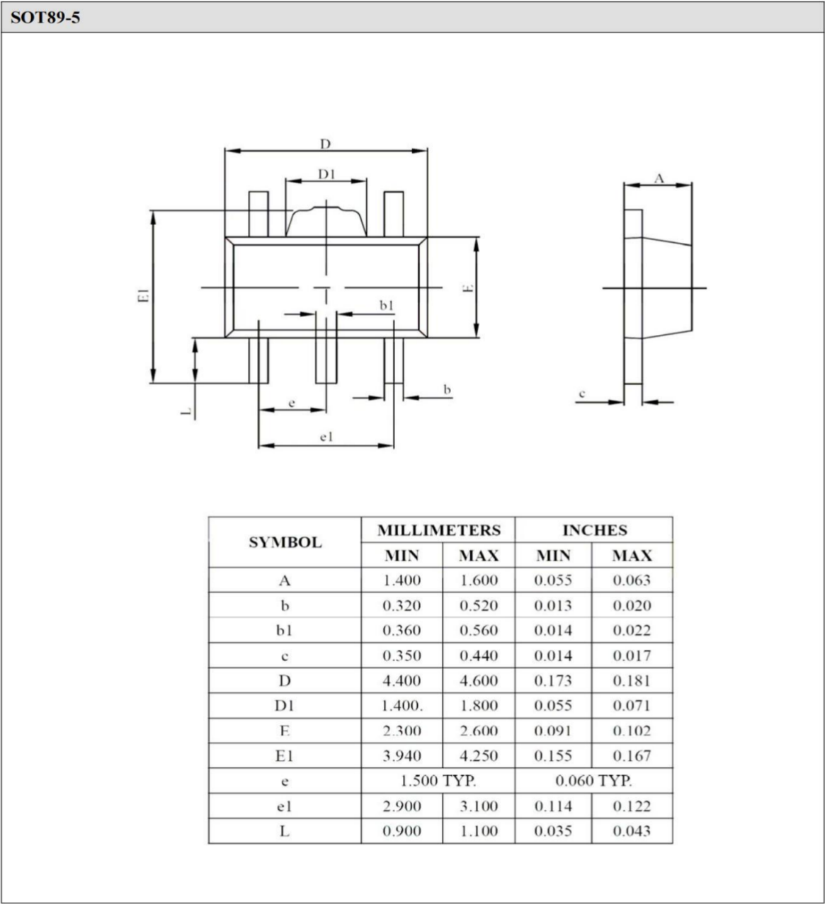
封装外形图:
