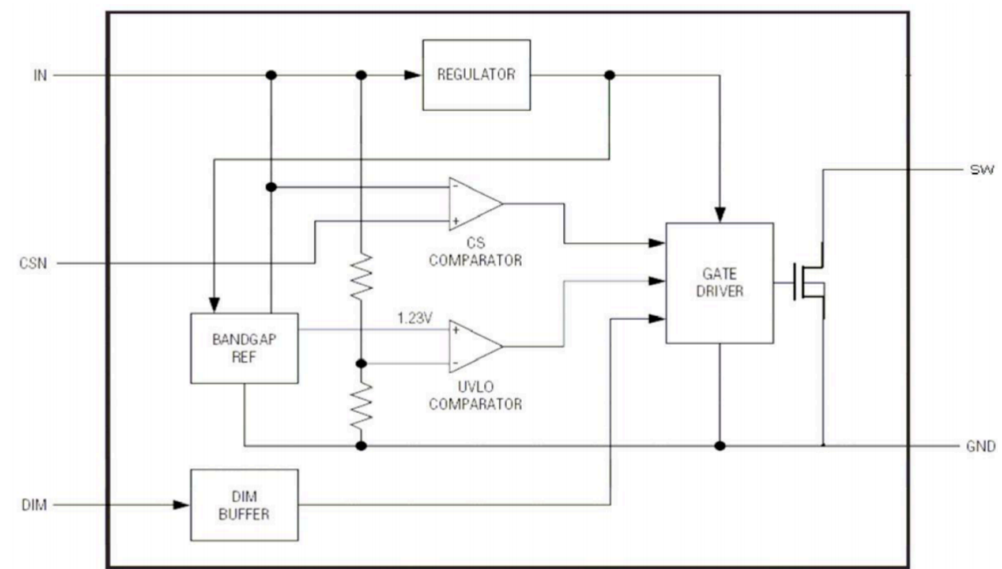
功能框图：
