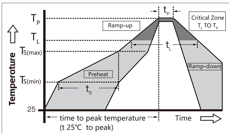
回流焊接参考温度 Recommend Reflow profile
