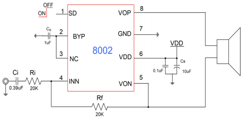
图 1 TD8002A 典型应用电路
