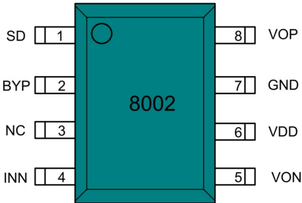
图 2 TD8002A 管脚定义
