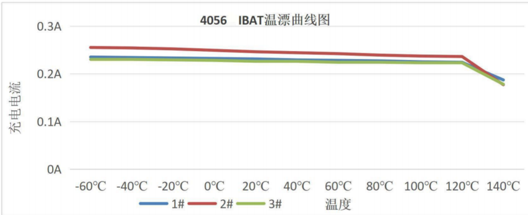
8.2 充电温漂曲线（VIN=5V，PROG=5.1K，ESOP8）
