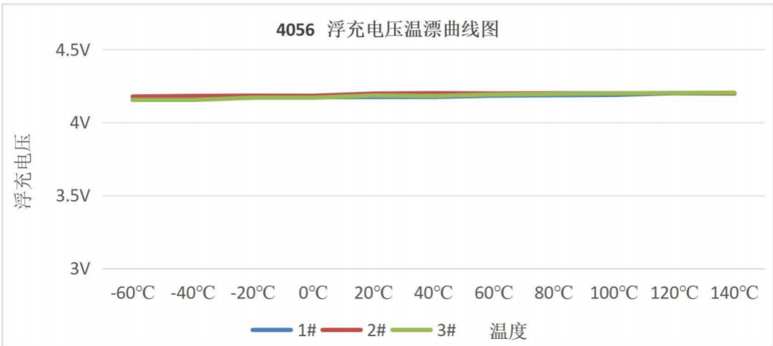
8.3 浮充电压温漂曲线（VIN=5V，PROG=5.1K，ESOP8）
