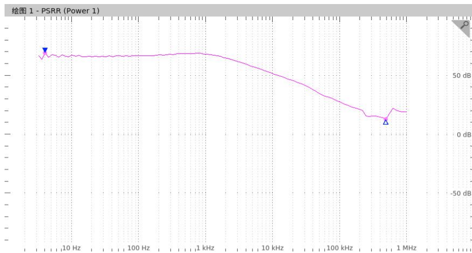
PSRR 曲线
