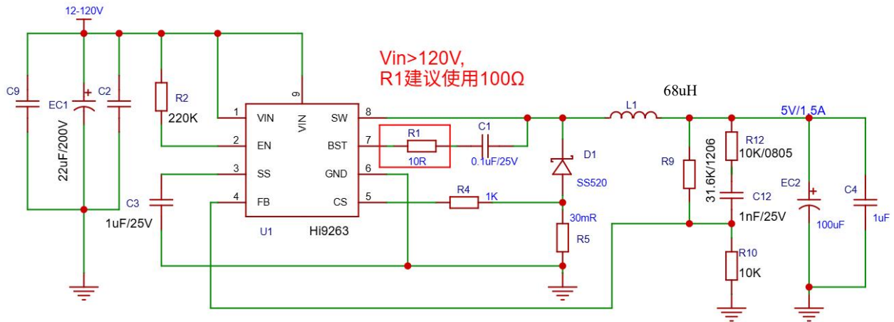
图三：Hi9263 输出 5V/1.5A 应用
