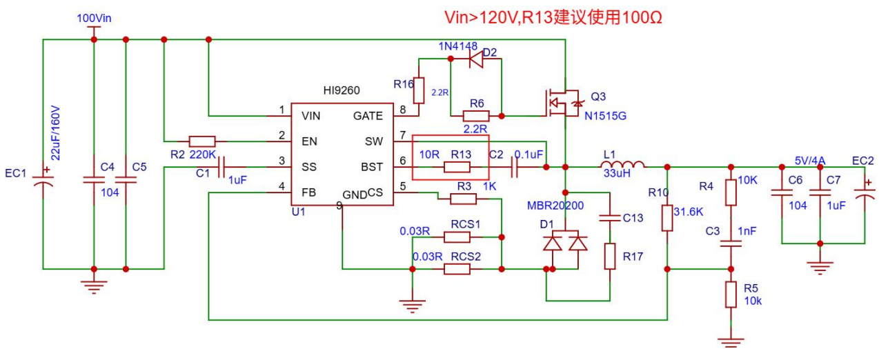
图四：Hi9260 输出 5V/4A 应用
