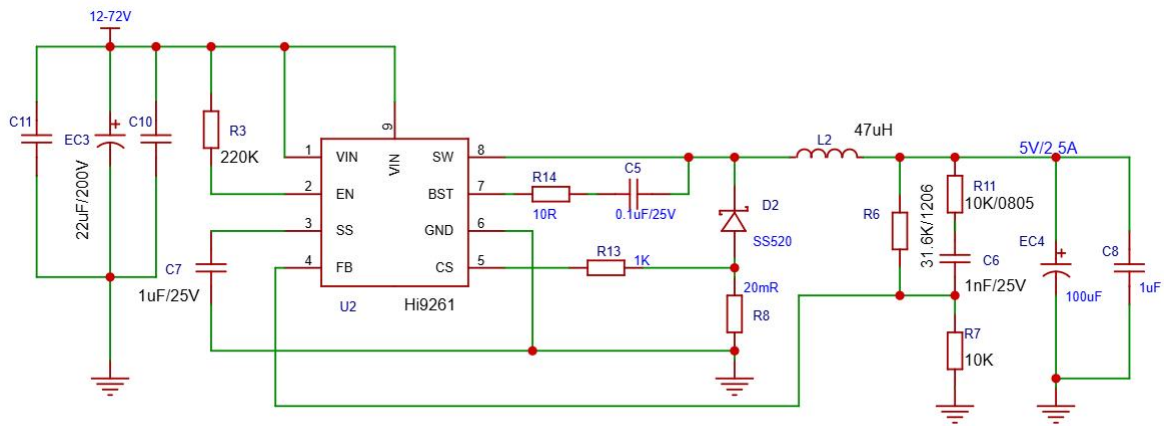
图三：Hi9261 输出 5V/2.5A 应用
