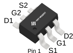
SOT-363 (SC-70-6)
