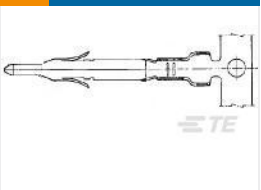
TE Part #170363-4 MINI UNIVERSAL M-N-L PIN LP
