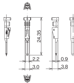
PQ50A-##PC#A
