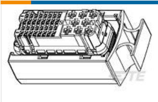
TE Part #368383-1 40P REC HSG ASSY(SIEMENS) BLK
