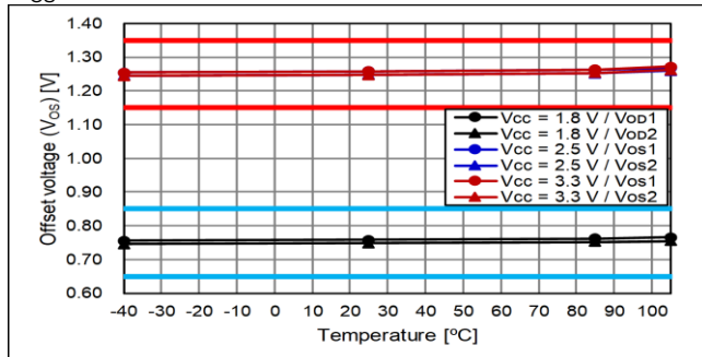
V OS
