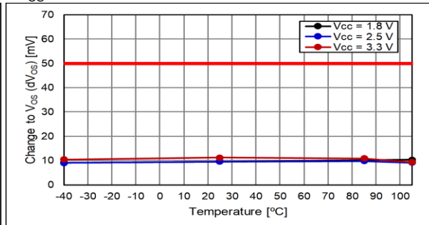
dV OS
