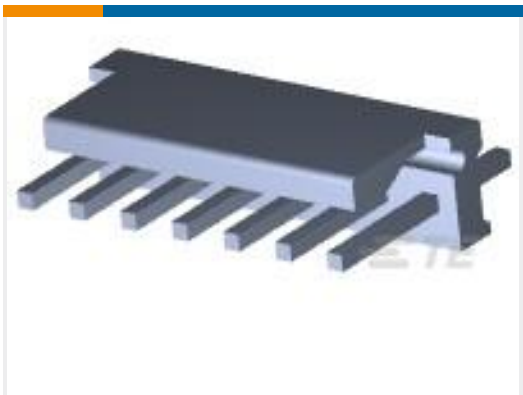
TE Part #644752-7 07P MTA156 HDR ASSY SQ STR F/L
