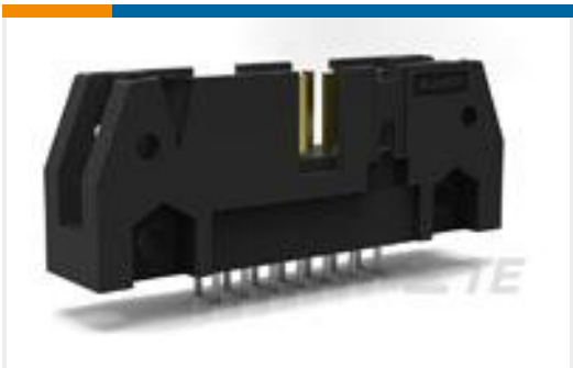
TE Part #5102153-8 A/L UNIV HDR 34P VERT
