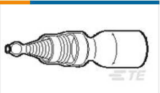
TE Part #705489-000 SGRS-1
